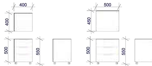
Откатная тумба
