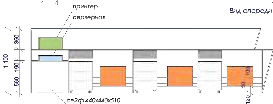
Вид изнутри
