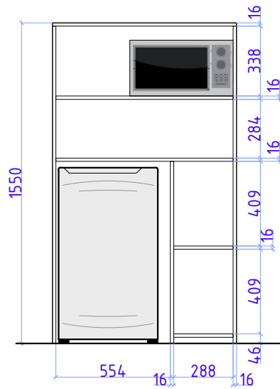
Разрез спереди
