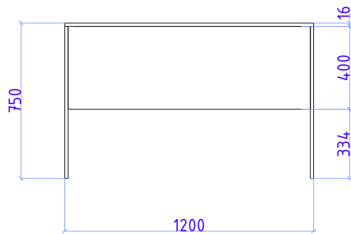
Вид спереди (1)
