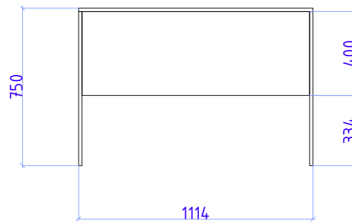
Вид спереди (2)
