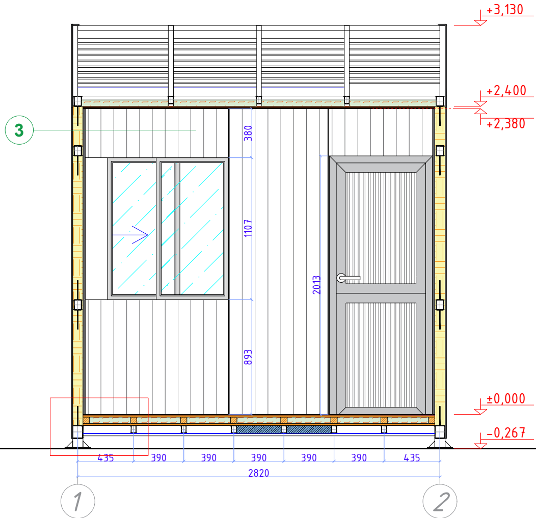
Разрез Б-1
